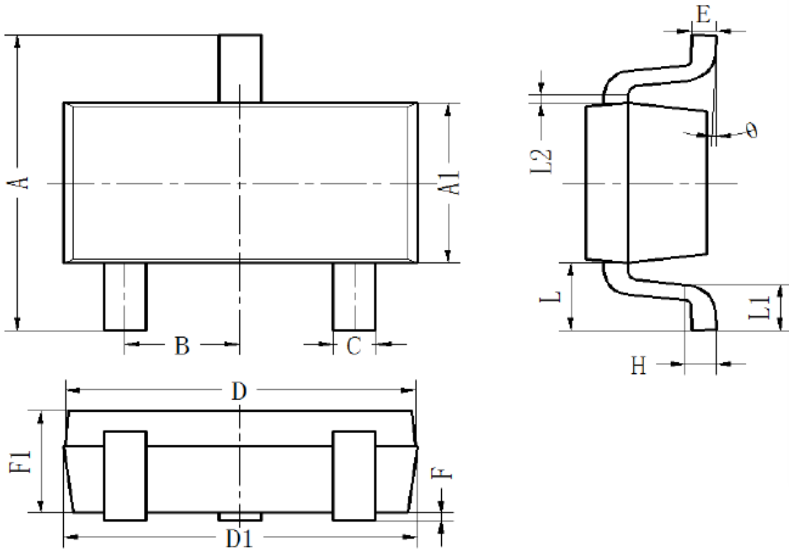
SOT 23-3
