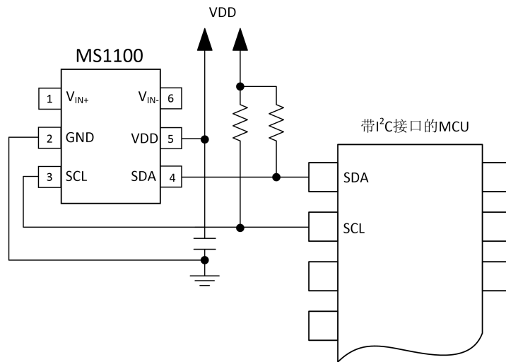
图 4. MS1100 的典型连接方法
