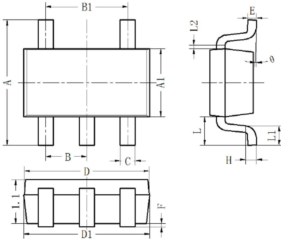
SOT23-5L
