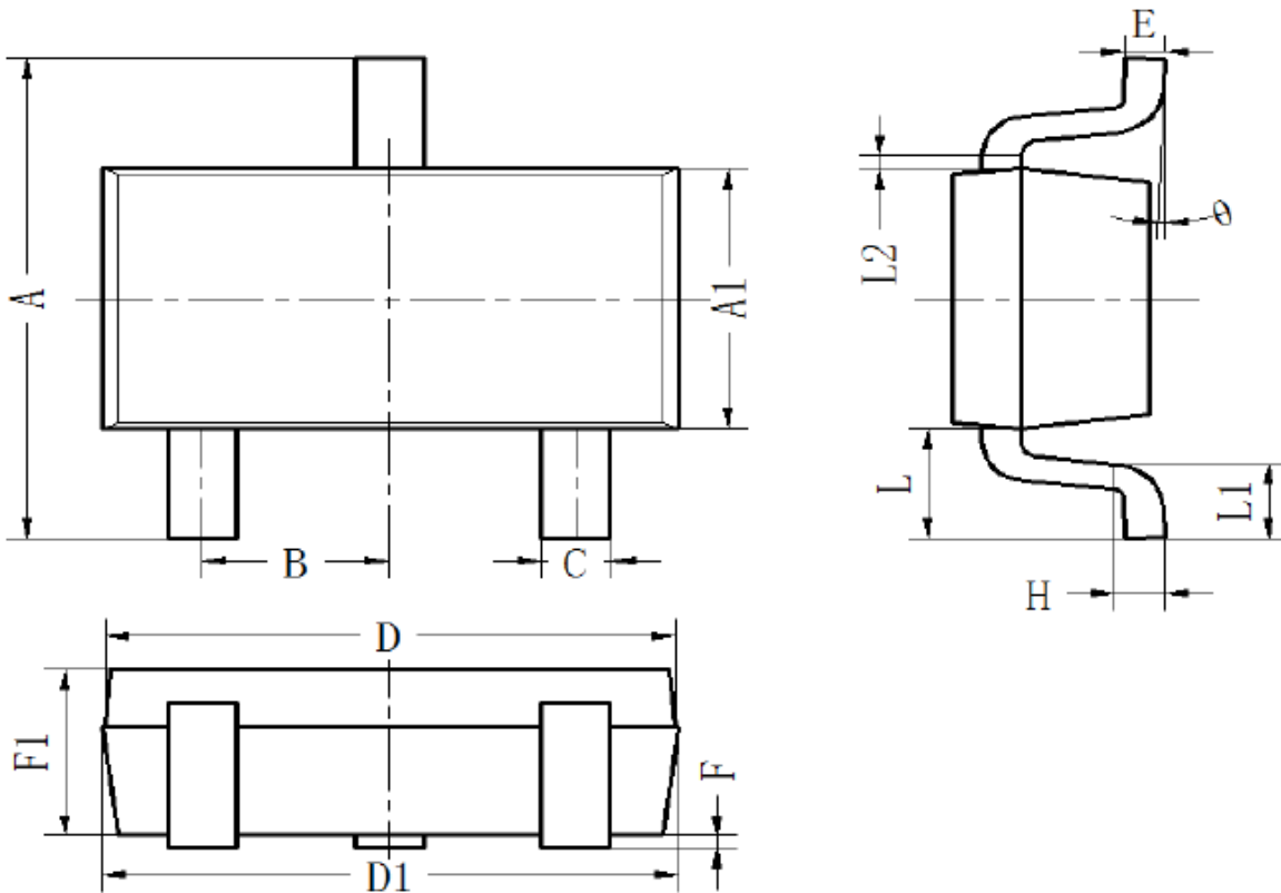
SOT23-3L
