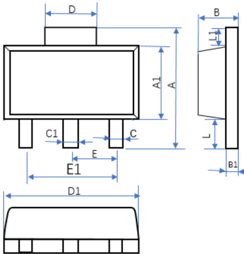
SOT89-3L
