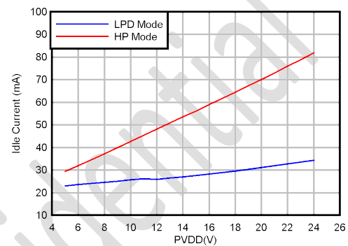
(Fsw=480kHz, LC Filter=10uH+0.68uF)
